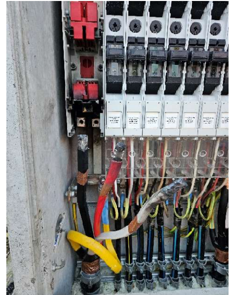
Kurzschluss an der Einspeisesiche- rungsleiste
